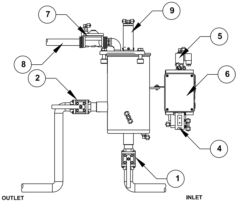
WITHOUT C.O.V.
